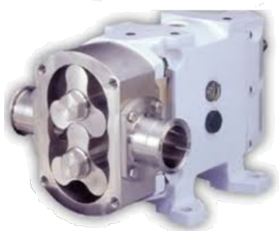
Sistema de dosificación viscosos con partículas solidas.
